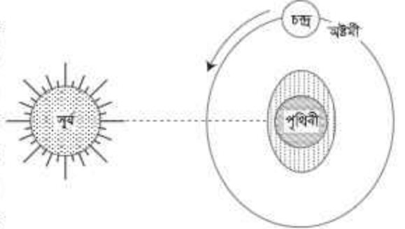
চিত্র ৩.১৪ : অষ্টমী তিথিতে মরা কটাল
